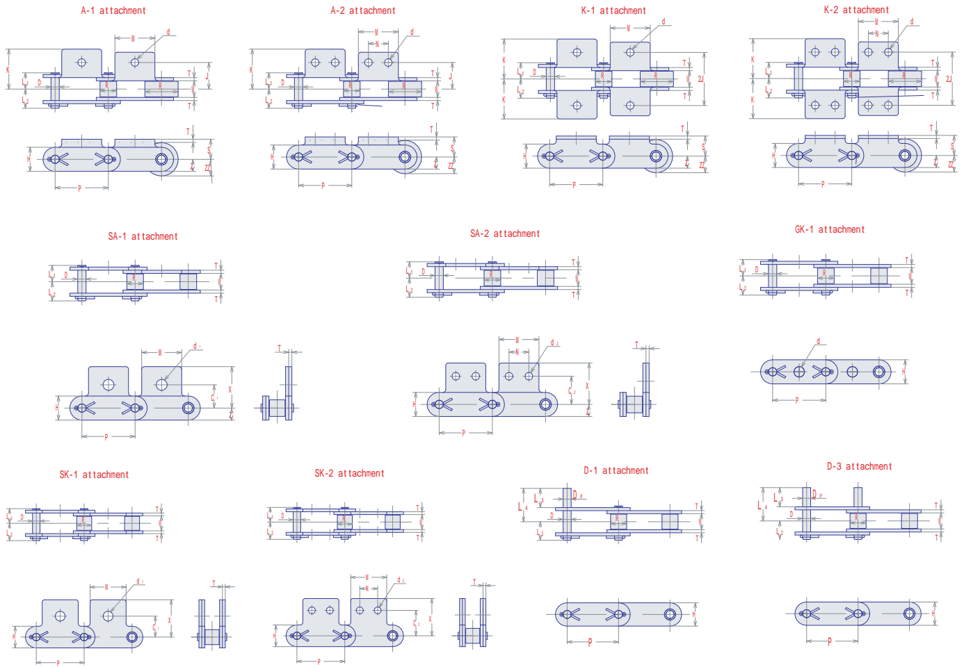
ダブルピッチローラーチェーンの基本仕様表
